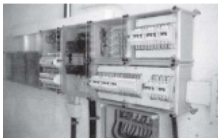
EL QUADRE ELECTRIC DEL COMPLEX ESPORTIU MUNICIPAL, UNA VEGADA MODIFICAT
